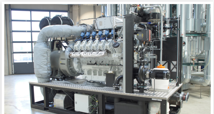
Neuentwickeltes Blockheizkraftwerk ECO 495 mit einer Leistung von 390 kW el
